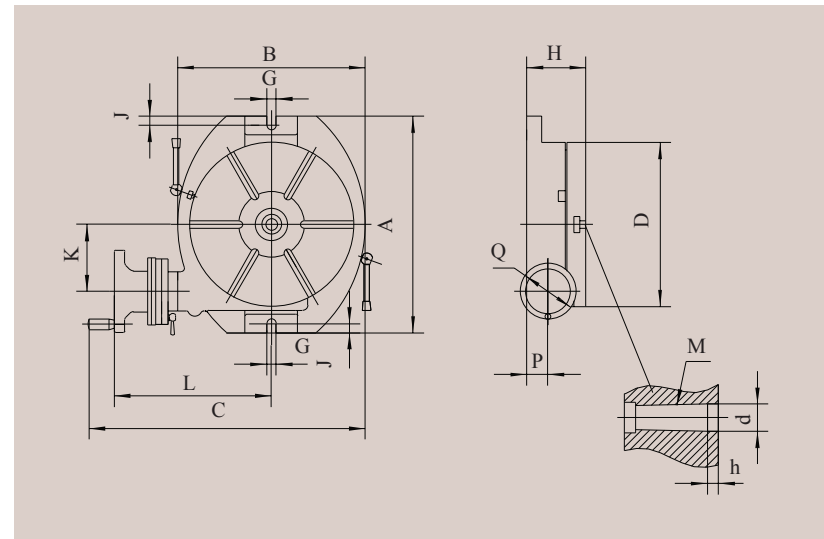
1001-0160...2500 ,1001 (TS) 系列回转工作台安装尺寸参数：Installation sketch and dimensions
